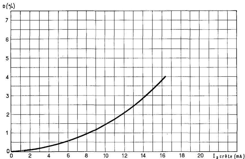
Fig. 5. — Distorsion totale D% en fonction de I_a (crête) pour le tube E 810 F Dispositif d'essai : amplif. sym. différentiel à contre-réaction. V_a = 110 V; V_{g2} = 120 V. R_{sa} = 1\ 200\ \Omega , R_k = 900\ \Omega (commune); V_{pol} = -42 V. I_a (.) = 2 \times 22 mA (équilibrés, avec alimentations séparées pour les deux polarisations).
