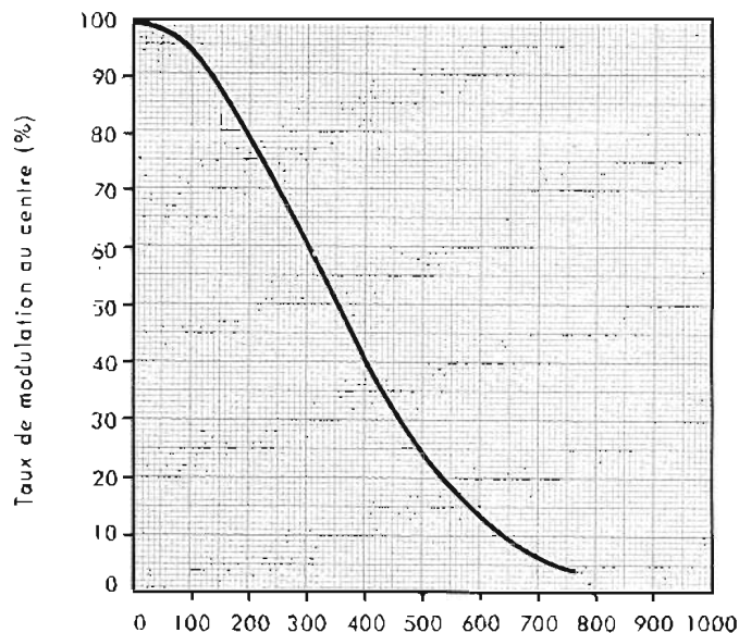
Fréquence spatiale (lignes TV)
