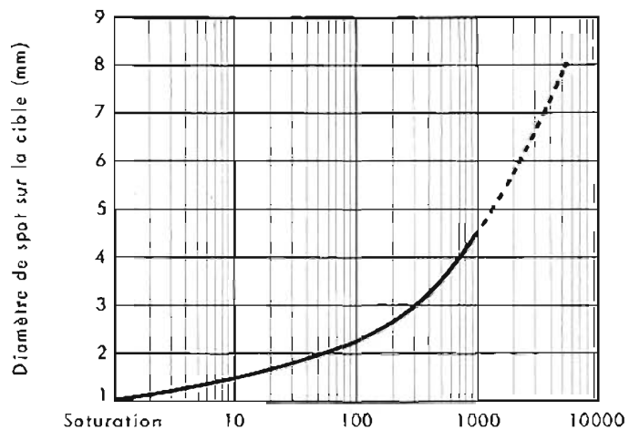
Niveau de lumière au dessus de la saturation
