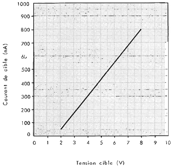
Figure 2 - Caractéristique de courant de cible de saturation.
