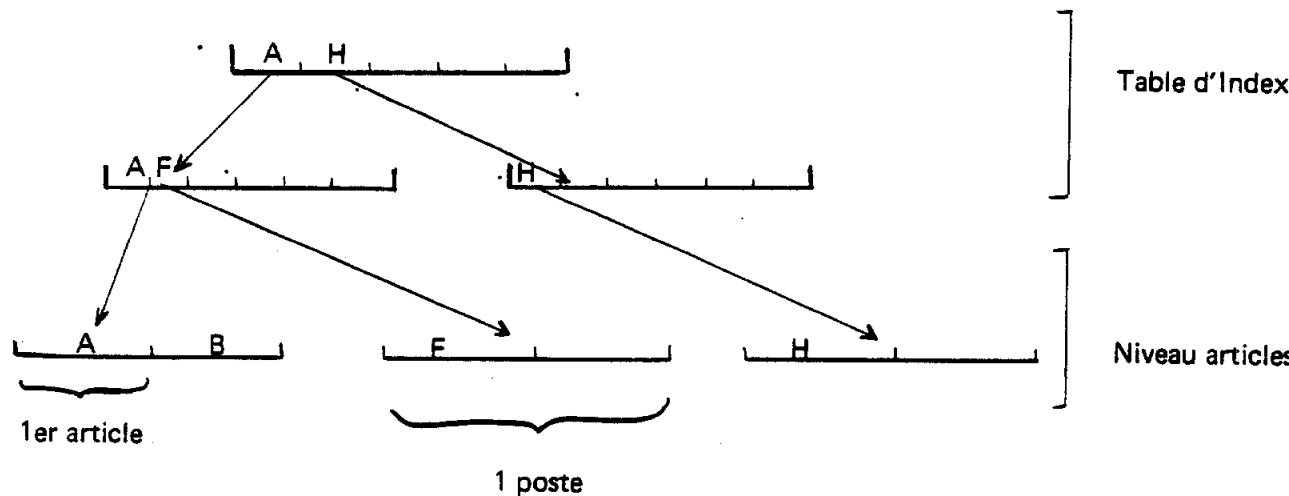
Structure arborescente d'un fichier Séquentiel Indexé
