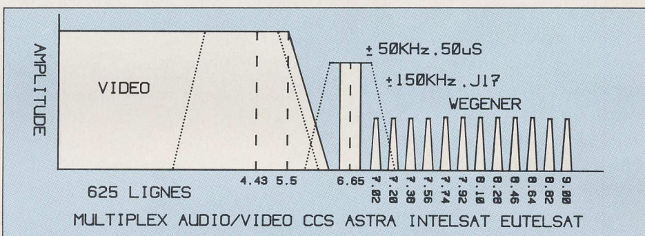
Fig. 3. - Spectre du signal d'un canal type ECS.
