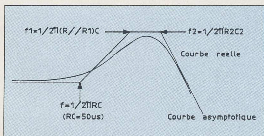
Fig. 6. Courbe de réponse du filtre.
