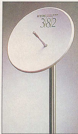
Antenne circulaire à guide d'onde TDK 3/8/2. Convertisseur-tête à l'arrière. Diamètre 38,8 cm, bande 11,7 à 12,5 GHz, poids 1,8 kg.
