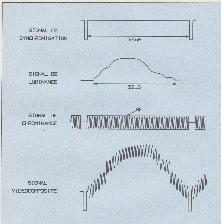
Fig. 1. - Composition du signal vidéo, somme de trois informations instantanées (PAL ou SECAM).
