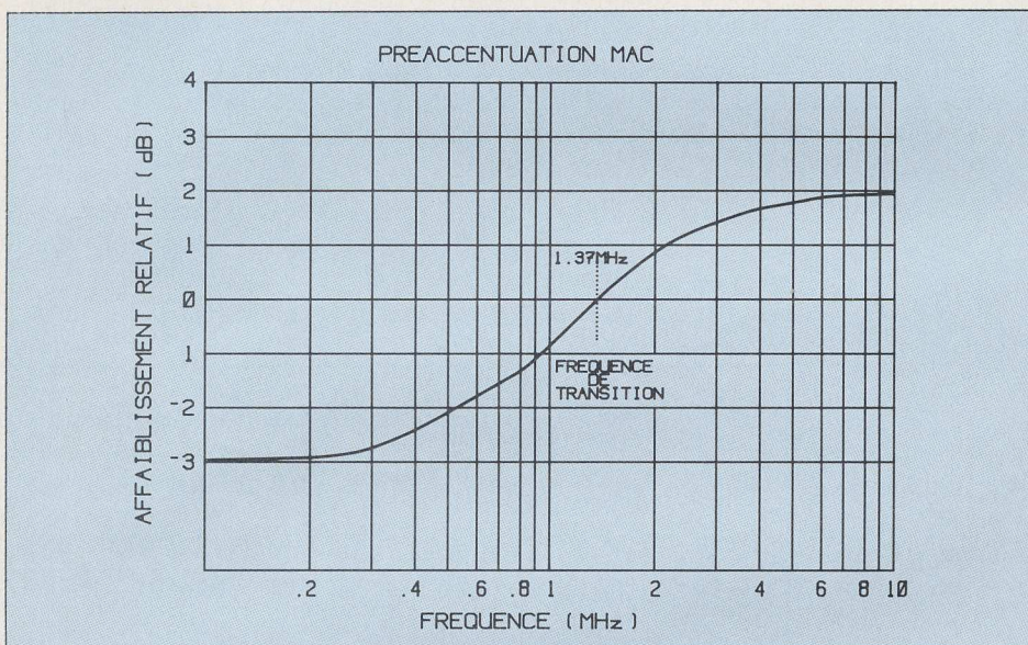
Fig. 8. - Caractéristiques de la préaccentuation vidéo dans le cas d'un signal MAC.
