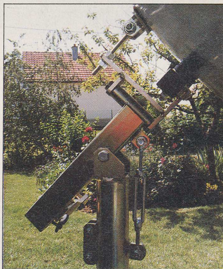
Une monture équatoriale sans son réflecteur. Les mécanismes d'inclinaison et de déclinaison sont bien visibles.
