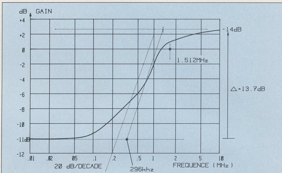
Fig. 4. - Allure de la préaccentuation selon la norme CCIR 405-1.
