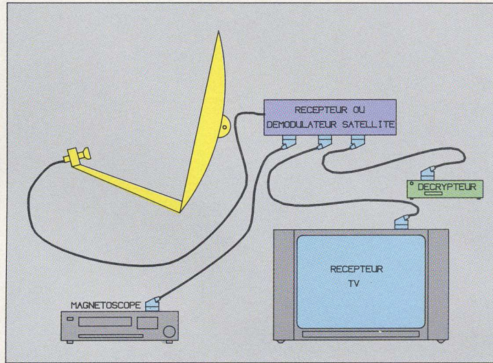
Fig. 2. Principe de connexion d'un décodeur avec un récepteur satellite à trois prises péritel.
