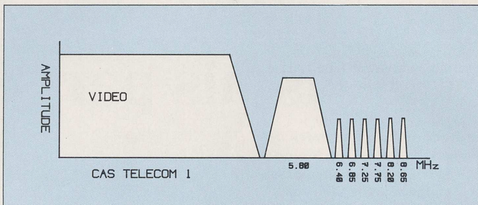
Fig. 2. - Spectre du signal d'un canal « Télécom ».
