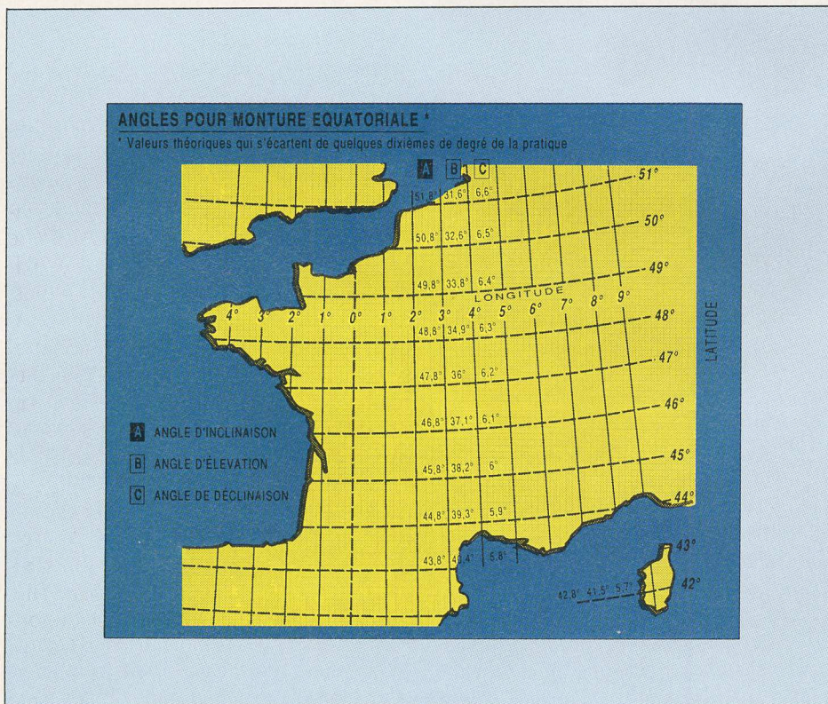
Fig. 2. - Angles de pointages pour quelques sites du territoire national.
