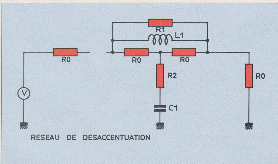
Fig. 9. - Structure de base du réseau passif.
