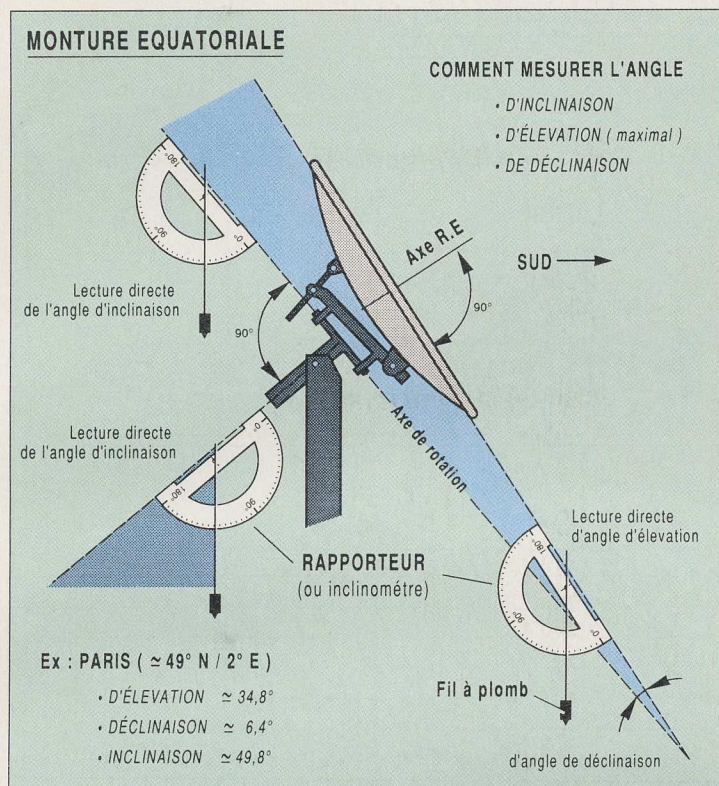
Fig. 3. Angles caractéristiques d'une monture équatoriale.
