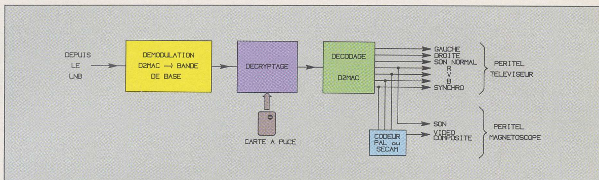
Fig. 1 Synoptique d'un décodeur/ décrypteur Eurocrypt.
