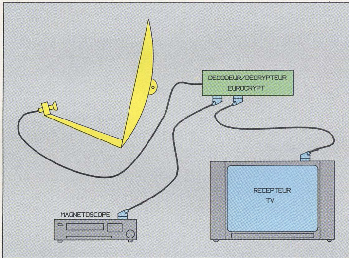
Fig. 3. Principe de connexion d'un décodeur Eurocrypt.
