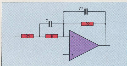
Fig. 5. Schéma du filtre de désaccentuation CCIR (audio).
