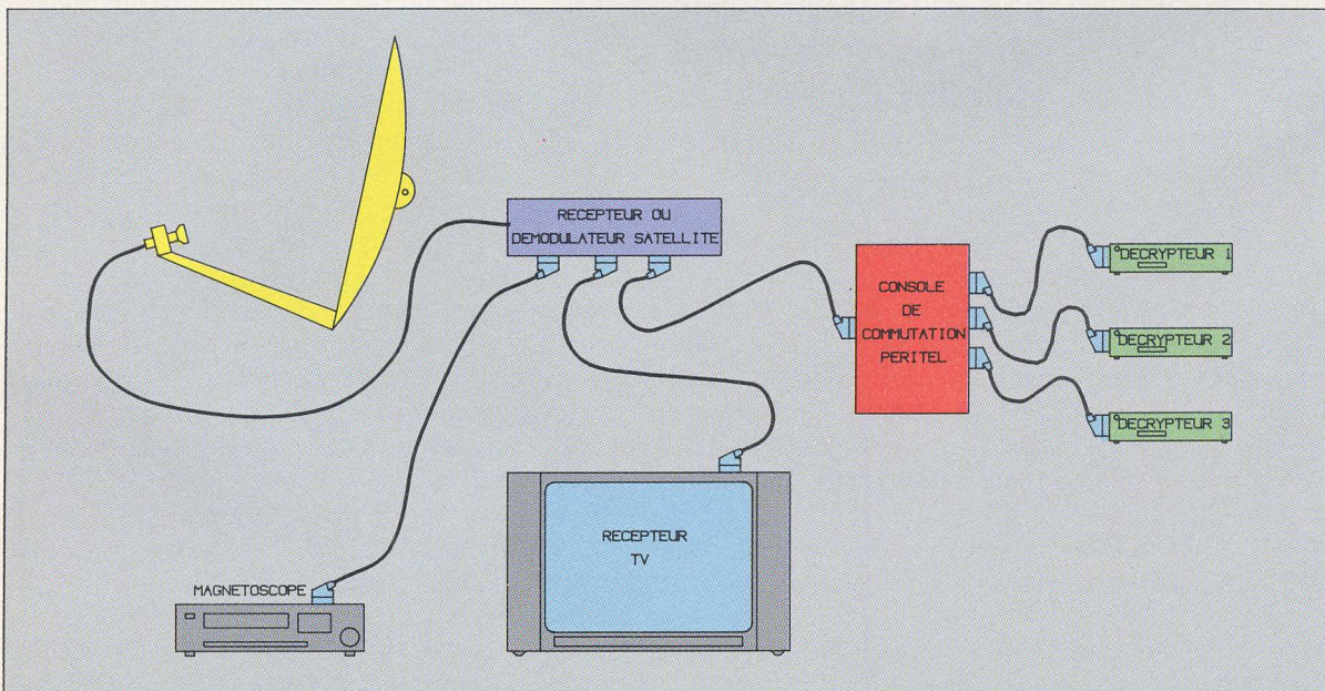
Fig. 4. Mise en place d'un boîtier de commutation lors de l'utilisation de plusieurs décodeurs.
