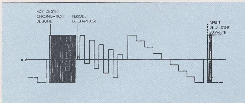
Fig. 7. - Composition d'un signal MAC, chaînage de données numériques et analogiques compressées.
