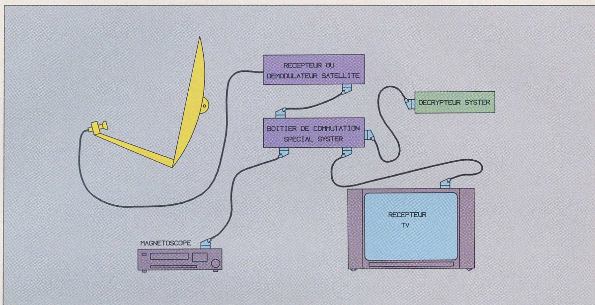
Fig. 5 Le câblage particulier à utiliser avec les décodeurs Nagravisystem de Canal Plus.
