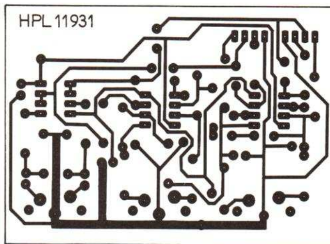
Fig. 2. — Circuit imprimé, coté cuivre échelle 1.
