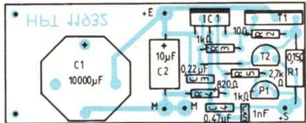
Fig. 3. — Implantation des composants.
