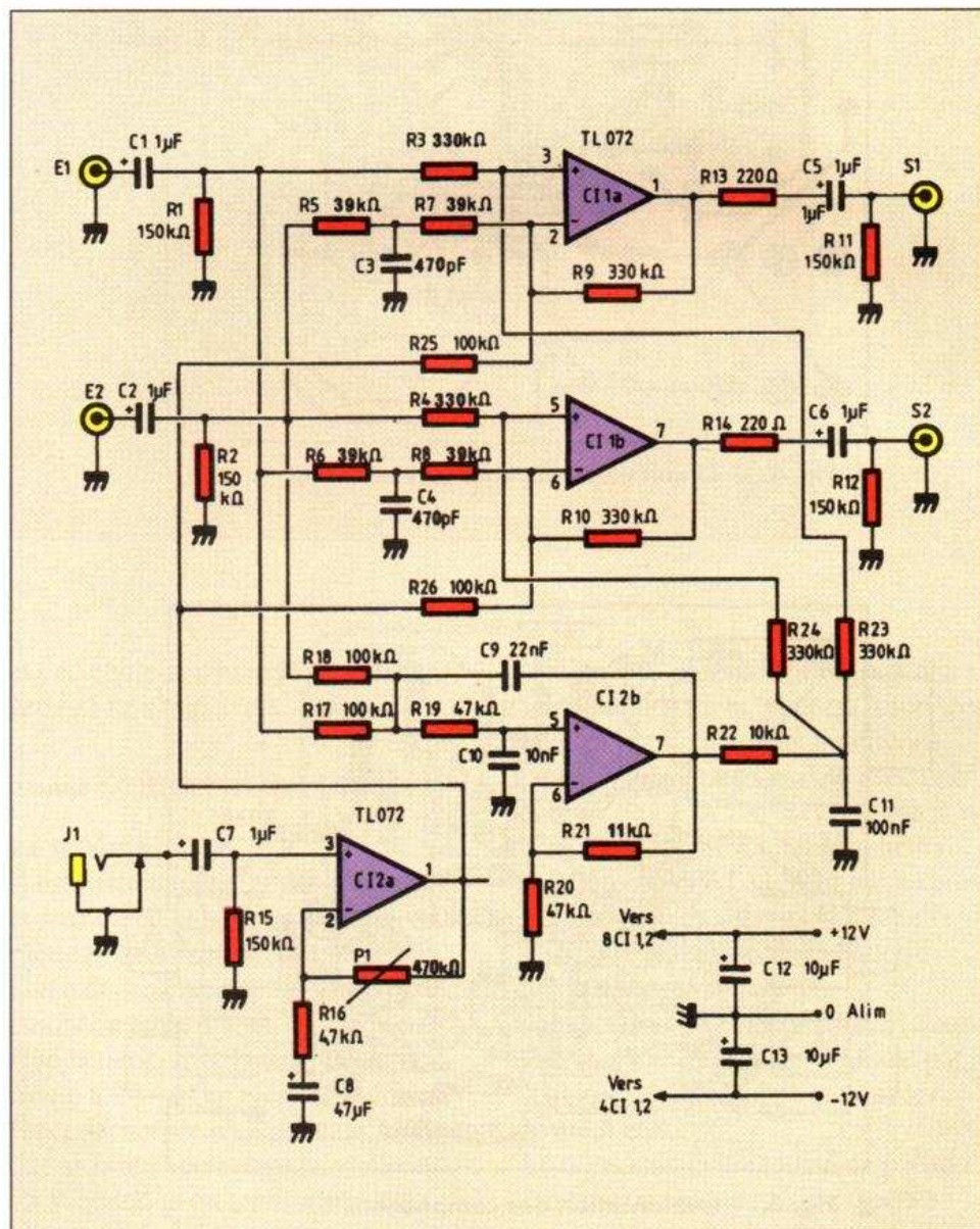
■ Fig. 1. — Schéma de notre montage.
