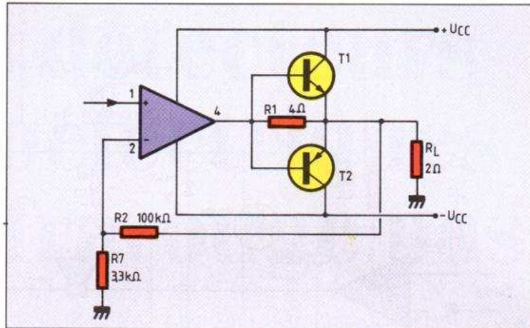
Fig. 13. — Au moment où l'un des transistors commence à conduire, un tiers de la tension fournie par la broche 4 se trouve déjà sur R_L .
