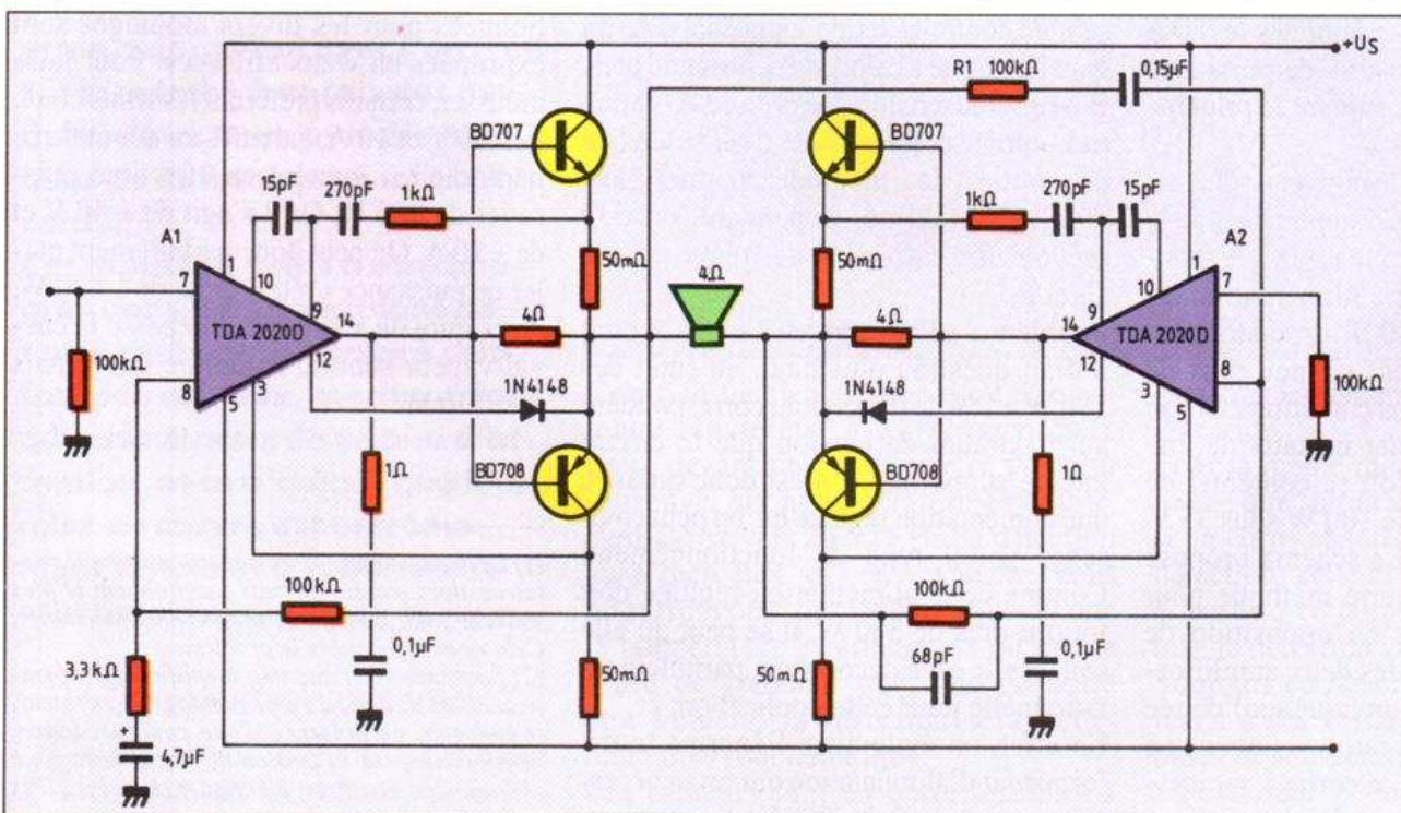
Fig. 14. — Avec deux amplificateurs fonctionnant sur le principe de la figure 12, on peut obtenir une puissance de 80 W dans une résistance de charge 4 Ω.
