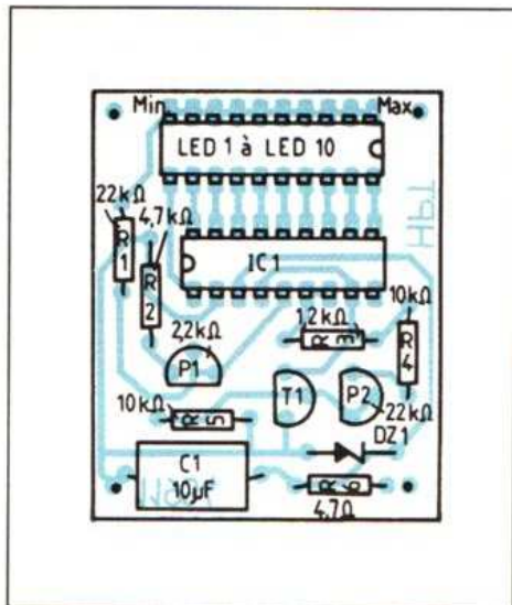
Fig. 3. — Implantation des composants.
