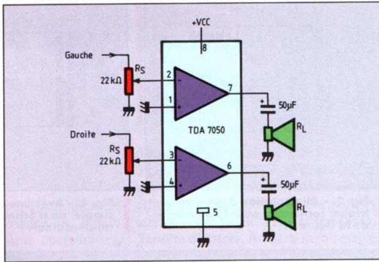
Fig. 7. - Amplificateur intégré de faible puissance, demandant un minimum de composants périphériques (schéma d'application Philips Composants).
