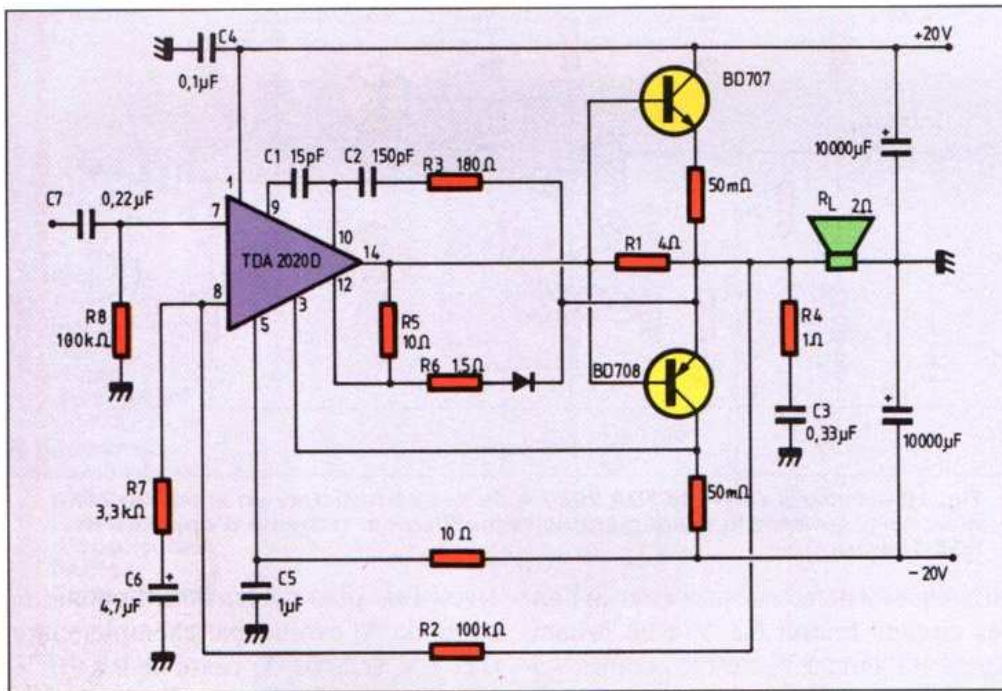
Fig. 12. – Utilisant les transistors supplémentaires en collecteur commun, on facilite leur protection mais on aboutit à un rendement médiocre.
