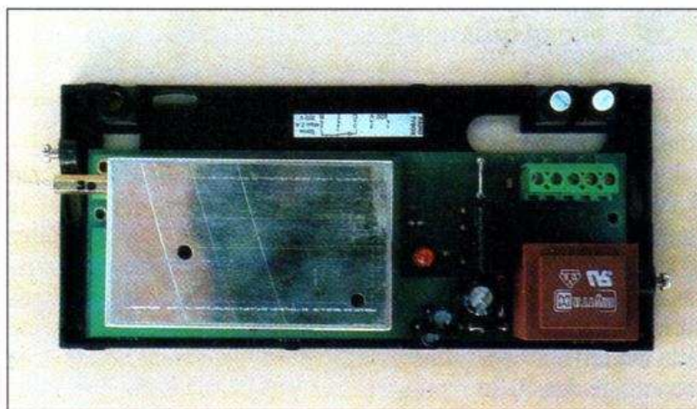
La partie haute fréquence du récepteur protégée par un généreux blindage.
