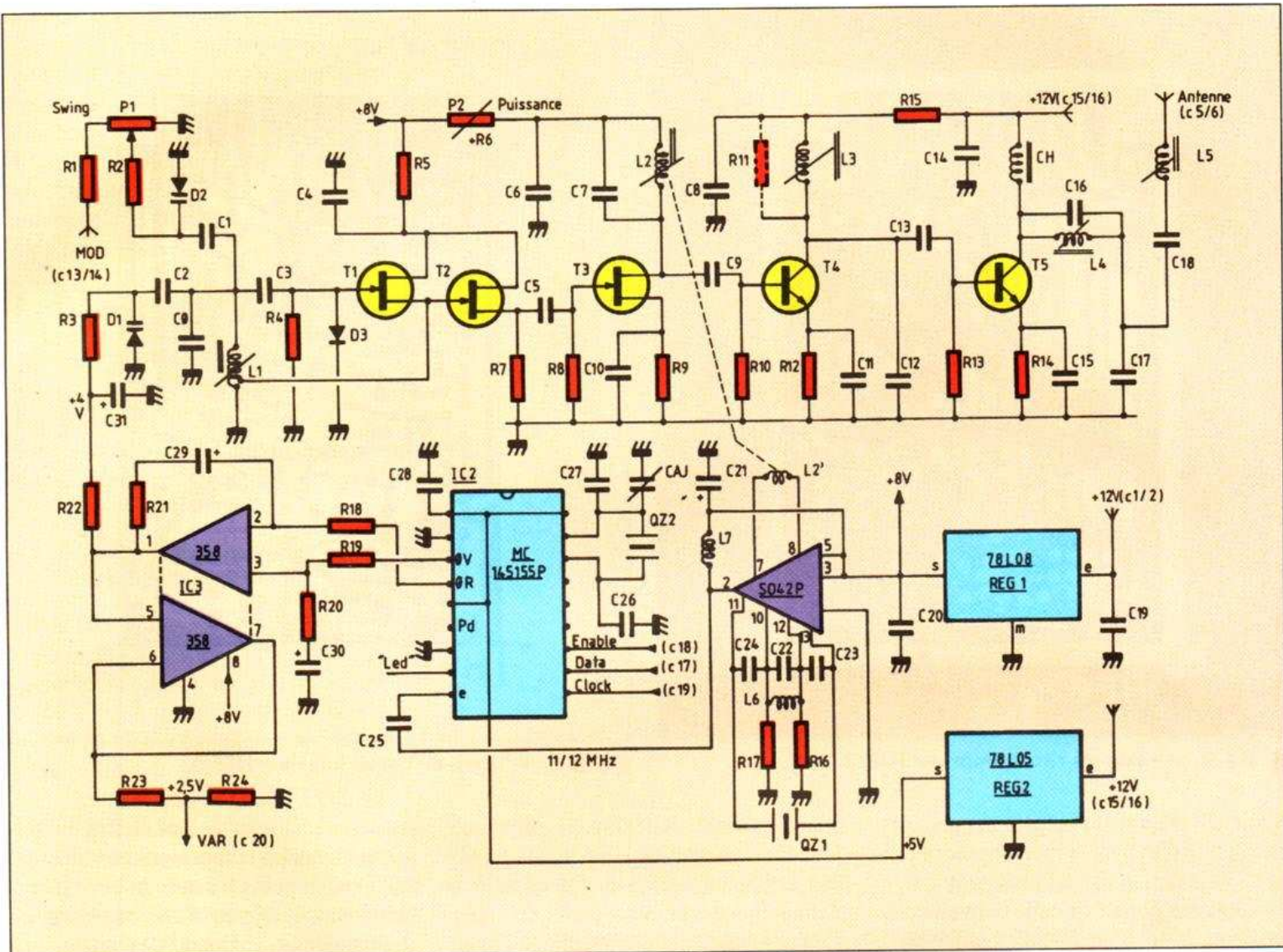
fig. 1. — Schéma de la platine HF8-SF/2.
