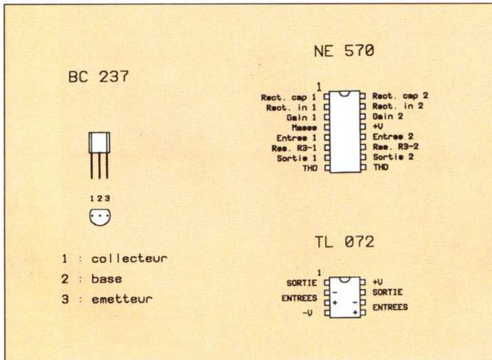
Fig. 5. — Brochages des principaux composants.
