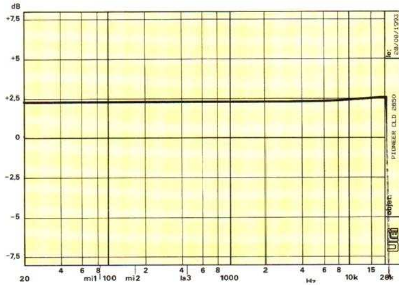
Courbe de réponse en fréquence en audio.
