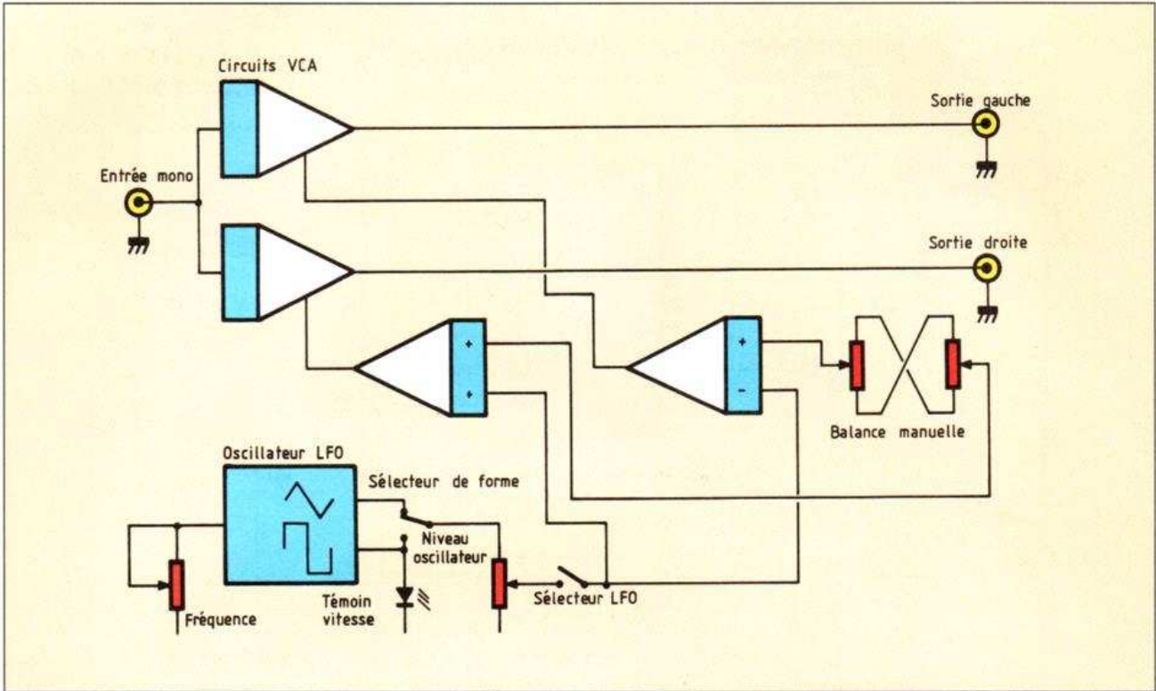
Synoptique du PN90.
