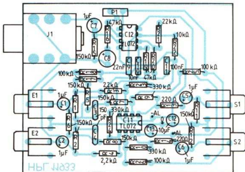
Fig. 3. — Implantation des composants.
