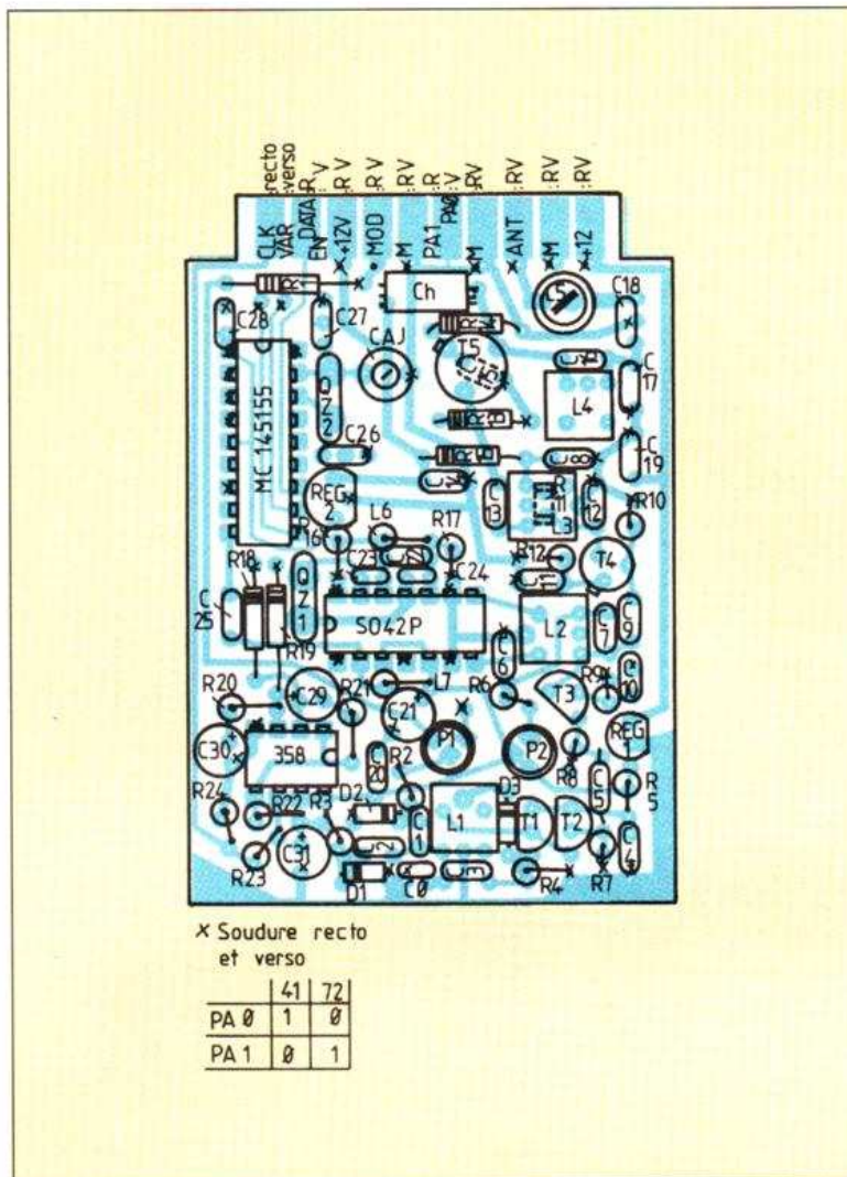
Fig. 4. — Pose des composants de HF8-SF2.
