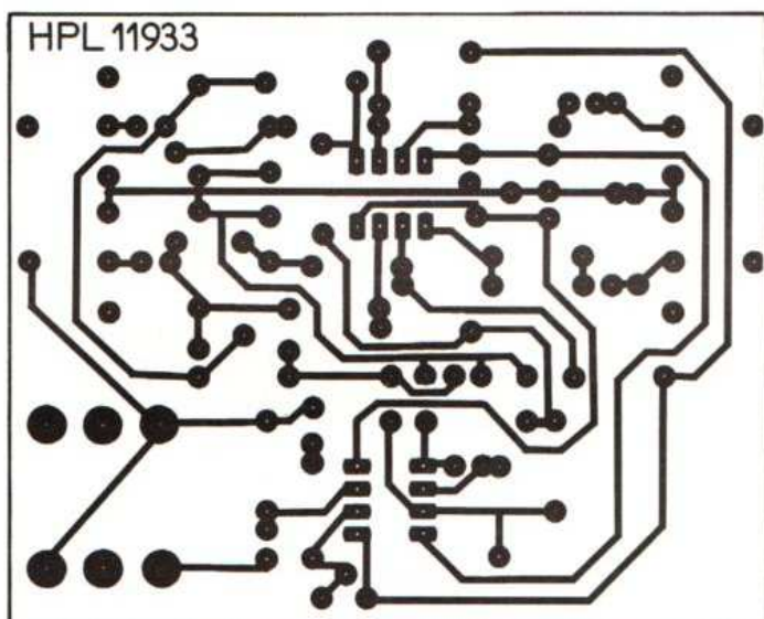
Fig. 2. — Circuit imprimé, coté cuivre echelle 1.
