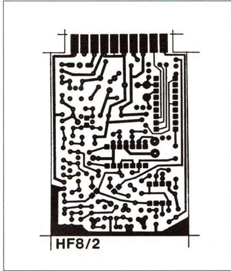
Fig. 3. — Verso du circuit imprimé HF8/2.
