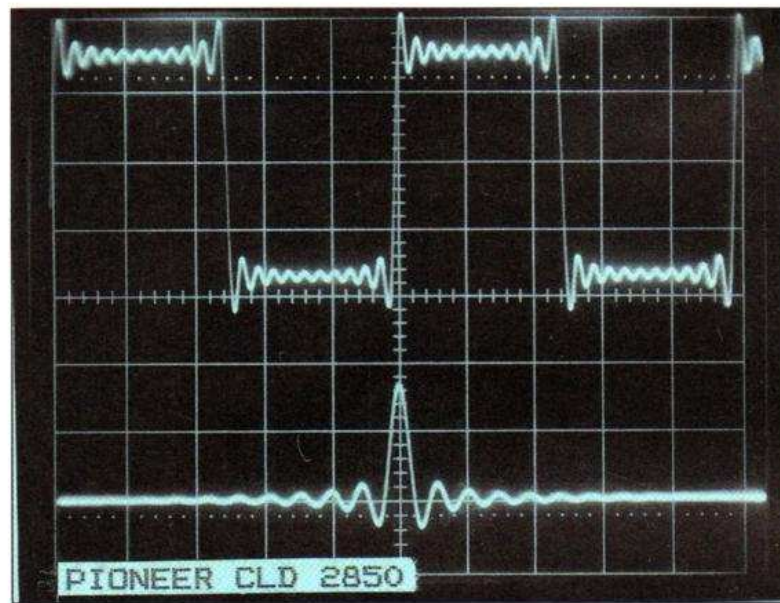
Réponse aux impulsions et aux signaux carrés.
