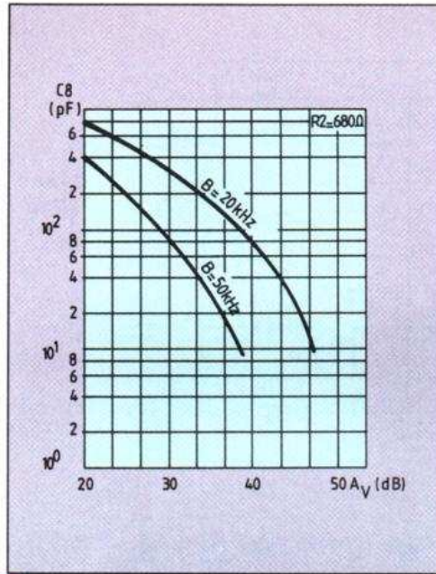
Fig. 2. - Graphique permettant de déterminer la valeur du condensateur C_8 de la figure 1.
