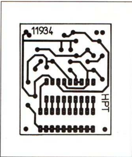
Fig. 2. — Circuit imprimé, vu côté cuivre, échelle 1.
