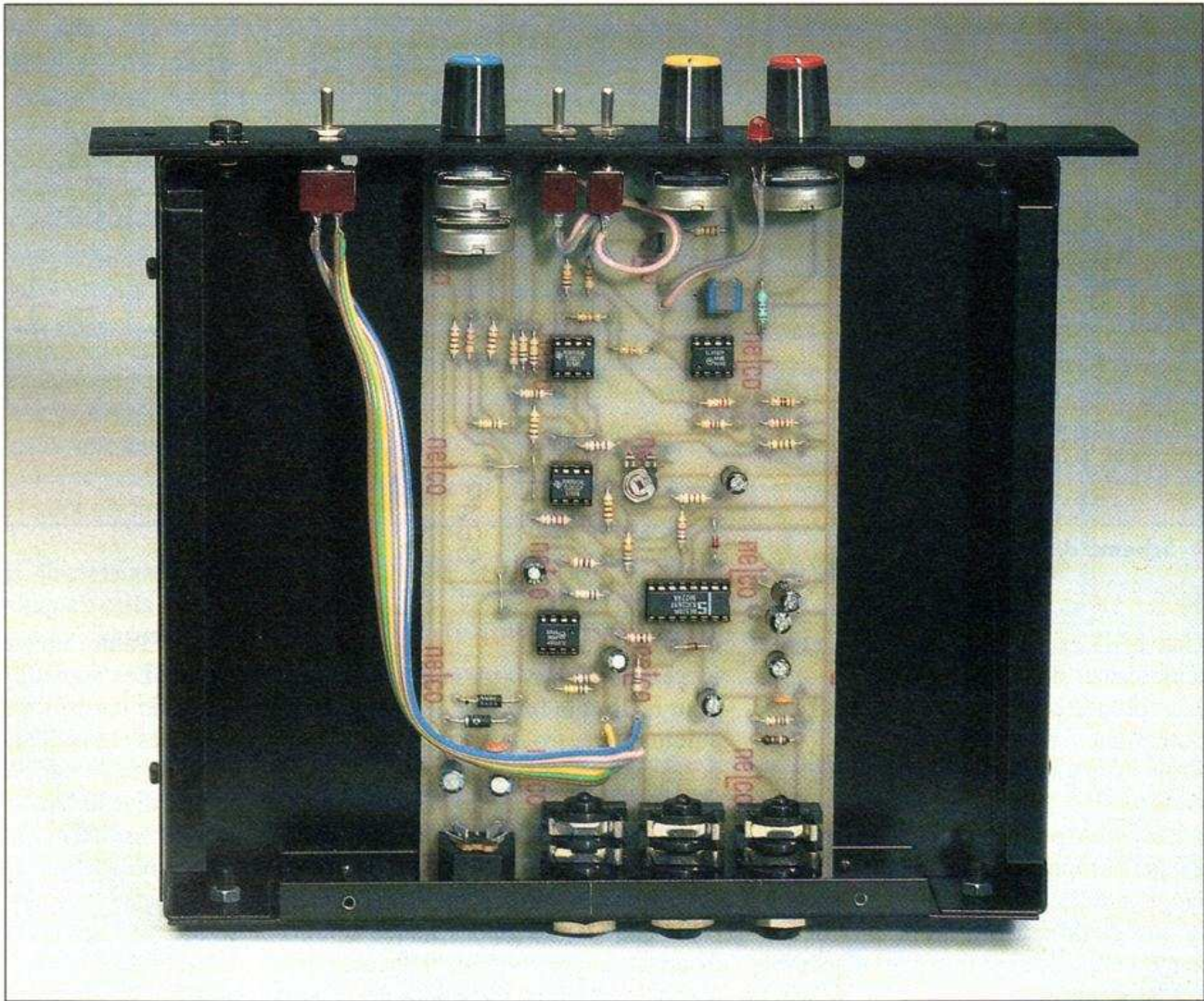
Vue de l'exécution interne du PN90.
