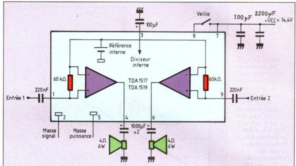
Fig. 9. - Amplificateur de moyenne puissance, à gain fixe, et se contentant de ce fait d'un nombre restreint de composants périphériques.
