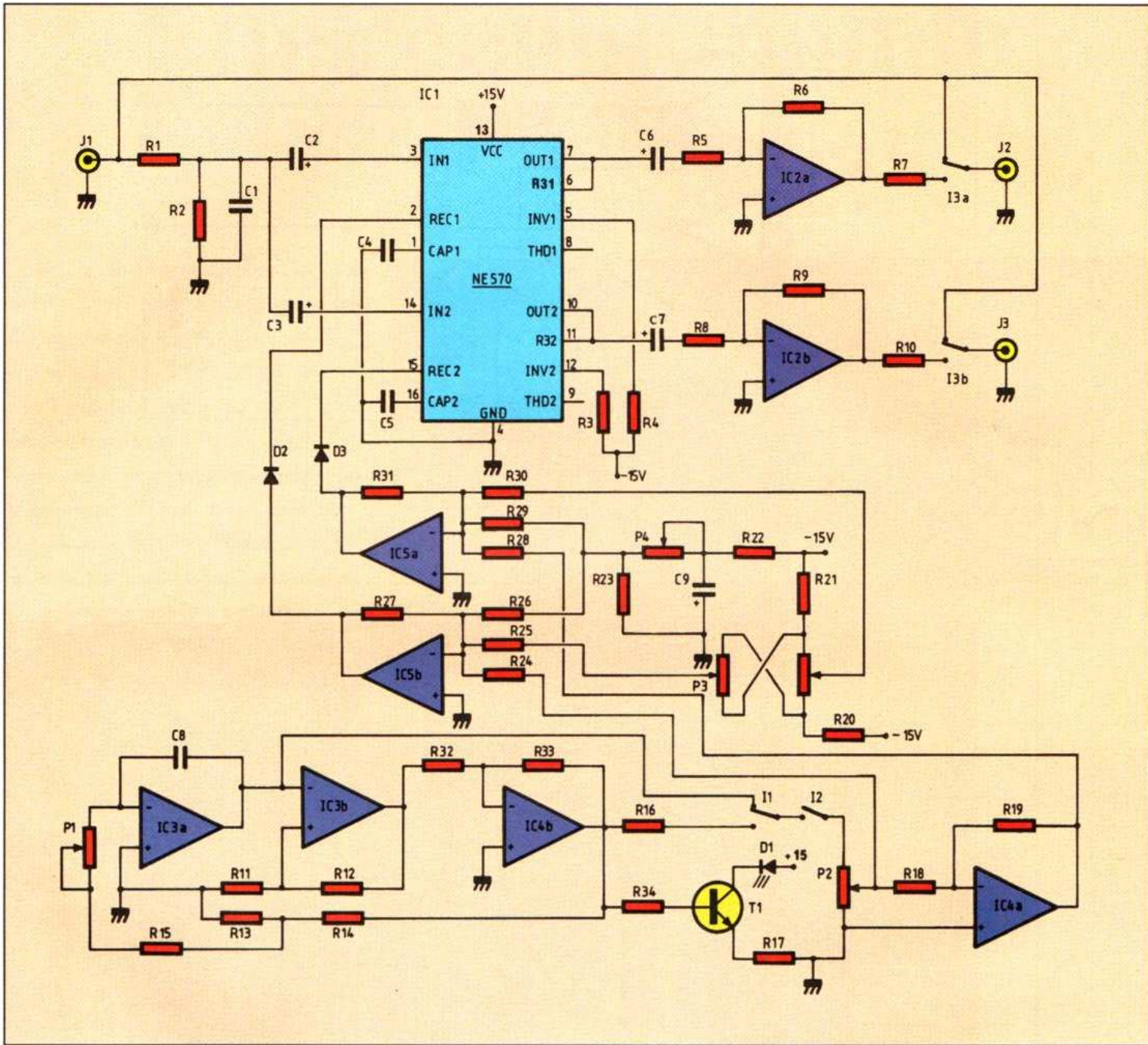
■ Schéma de principe du PN90.
