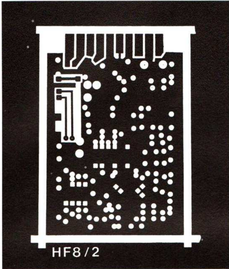
Fig. 2. — Recto du circuit imprimé HF8/2.
