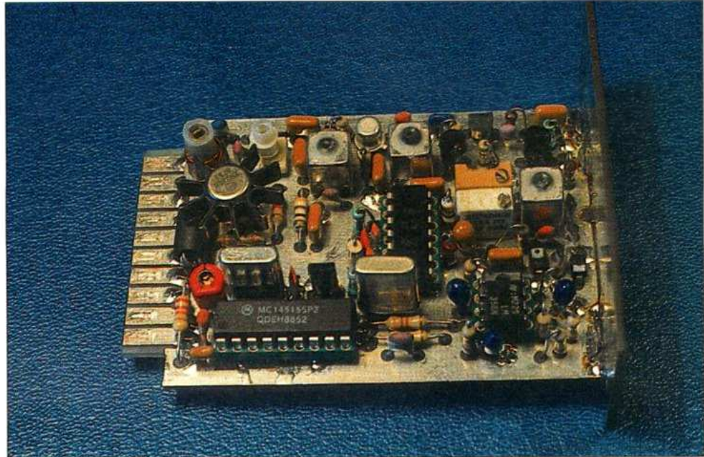
■ La platine HF8-SF/2 vue côté QZ1 et QZ2.
