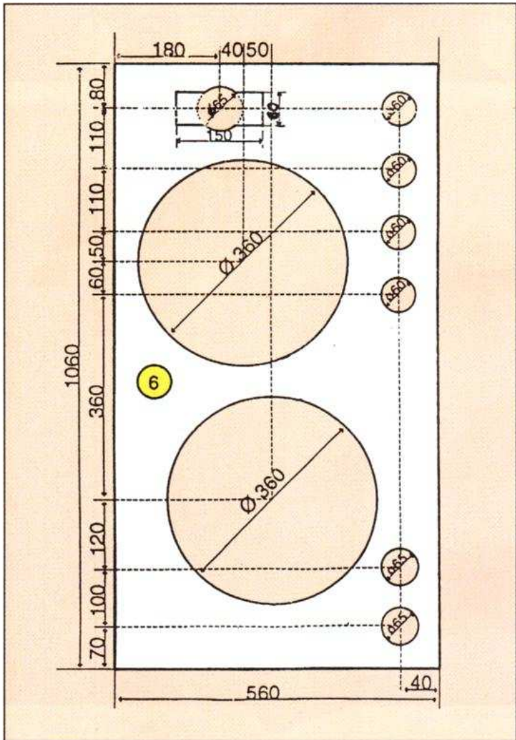
■ Diamètres des perçages de la face avant.
