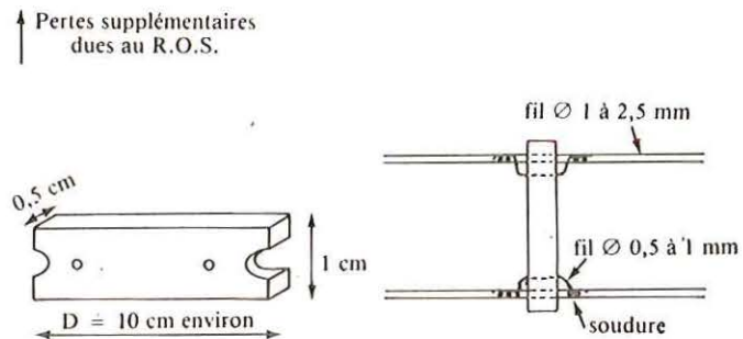
Fig. B.4.4a. Isolateurs à réaliser en matière plastique, luciflex ou plexiglas et méthode de fixation sur les deux fils de la ligne.
