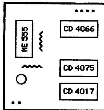
Figure n° 18 — Implantation des circuits du commutateur électronique.
