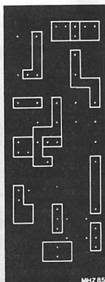
circuit imprimé du mélangeur
