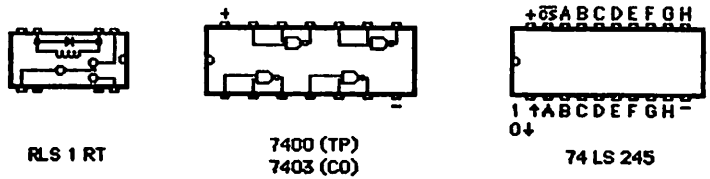
Fig. B : Schéma de l'alimentation - brochage des C.I. - adressage registre de contrôle du 8255.
