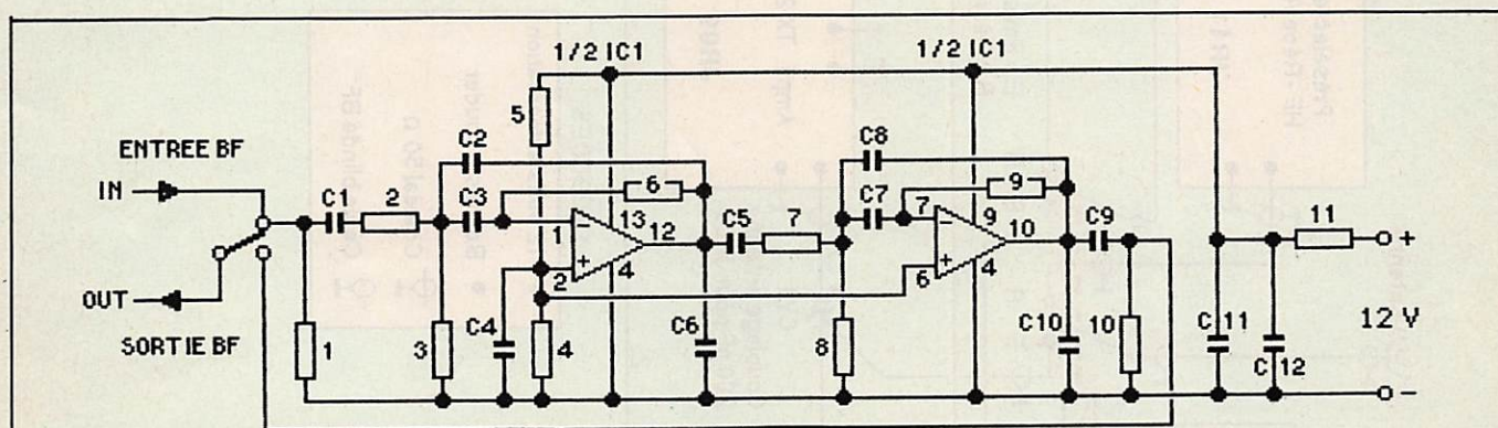
Figure 3 : Indicateur de puissance relative 302
