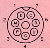
Brochage du connecteur 8 points des micros ADONIS.
