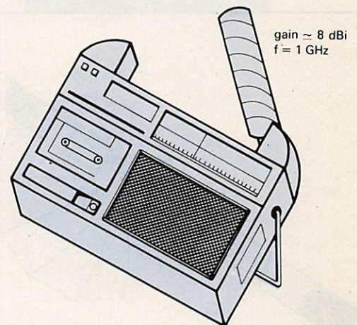
Figure 3 : Récepteur portatif avec antenne hélicoïdale
