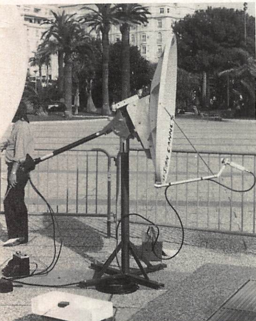
Vue d'ensemble d'une parabole offset 1. 20 m MASPRO motorisée.
