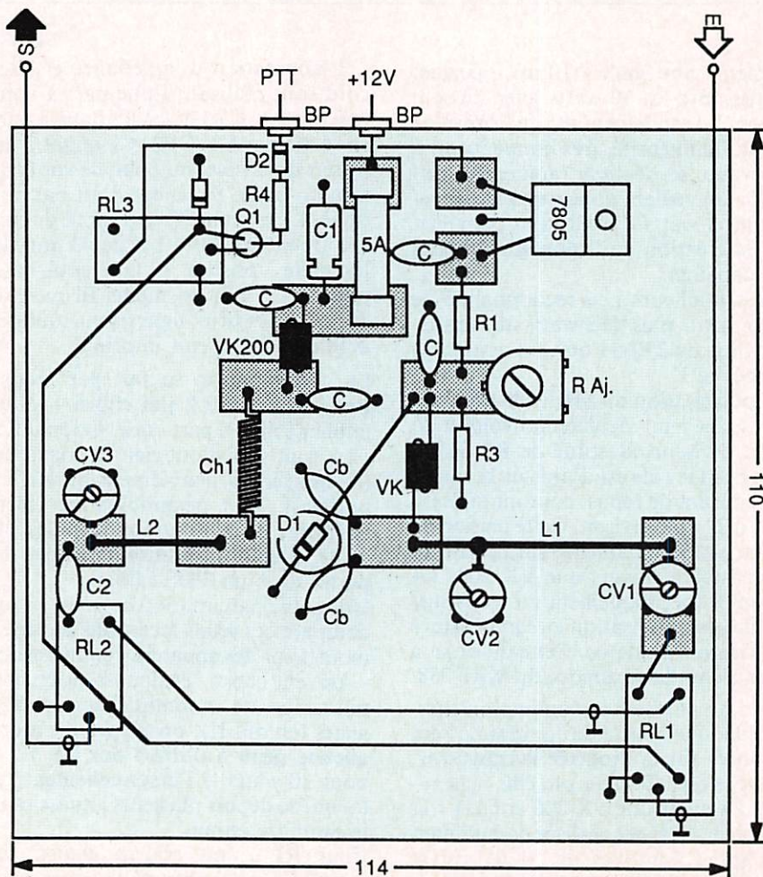
Figure 3 : Implantation des composants
