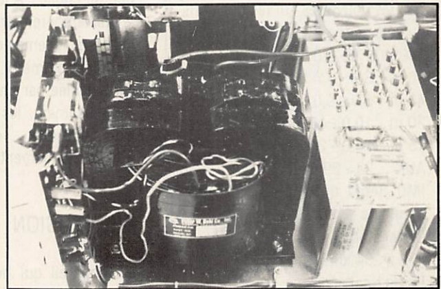
Le transfo en place. A droite, le pont de diodes, au-dessus des chimiques.
