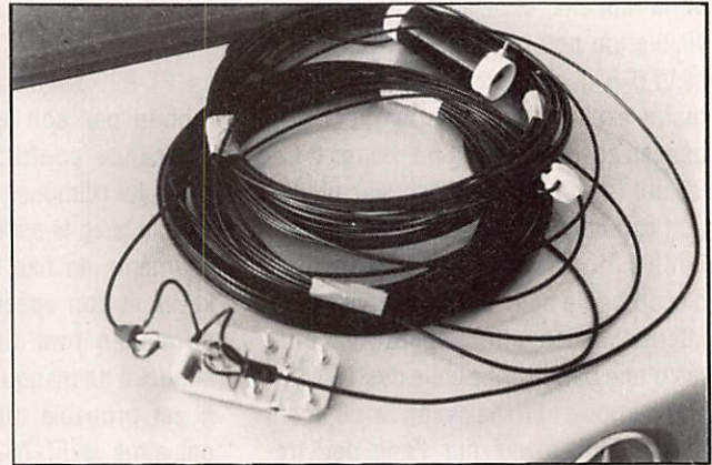
Arrivée du câble antenne sur une SO-239 attaches renforcées.
