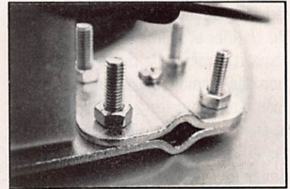
Fixation au pylône par écrous prévus d'origine.
