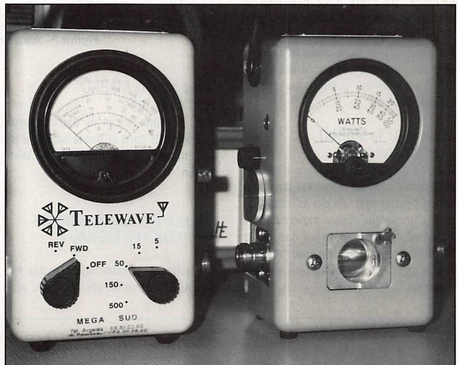
Photo A - Vue de face. A gauche : le Telewave équipé d'un commutateur de gamme de puissances et d'un commutateur de Pdir (FWD) et Pref (REV). A droite : le Bird dont le bouchon de mesure est enlevé, on aperçoit la ligne de transmission (âme).
