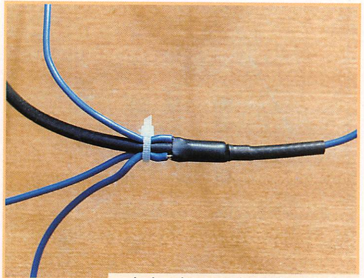
La jonction entre les radiaux, le brin rayonnant et le coaxial.
