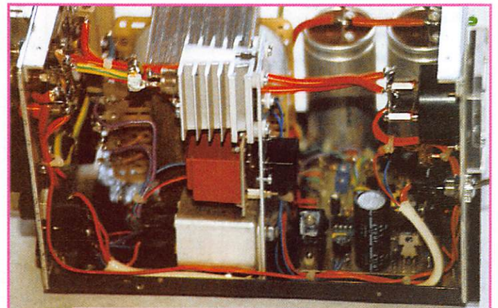
L'alimentation 24/28V vue de côté. On voit au centre le radiateur du thyristor qui est isolé du support, le TR2 monté sur un CI succinct, le filtre secteur et au fond à droite les 2 caps de 10 000 µF.
