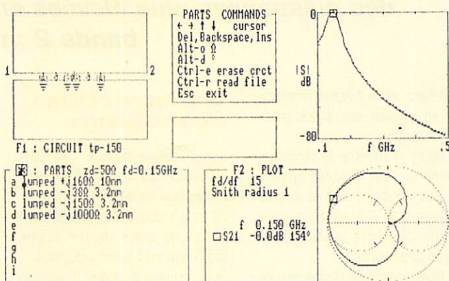
Fig. 6 : Recopie d'écran des caractéristiques des filtres obtenues avec le logiciel PUFF.
