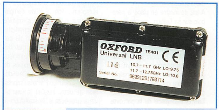
Une tête universelle avec commutation d'OL.
