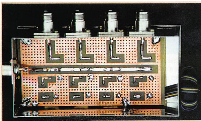
Vue de dessous de la platine à relais.
