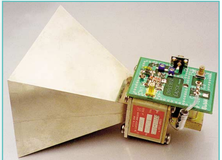
Un montage original utilisant un oscillateur-mélangeur à diode Gun.
