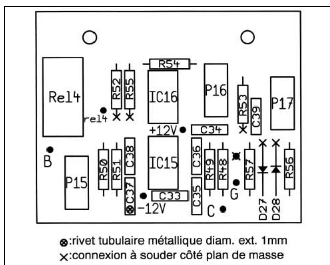
Circuit imprimé complémentaire : Implantation des composants.
