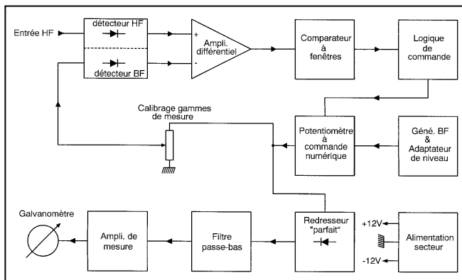
Figure 1 : Synoptique du millivoltmètre HF.
