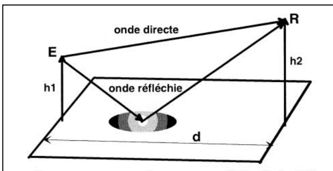
Fig.4 : Onde d'espace.
