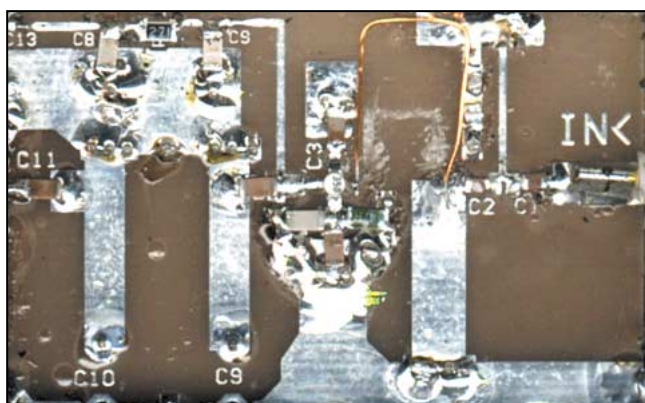
Photo 6 : Modification FILVO pour améliorer le facteur de bruit.
