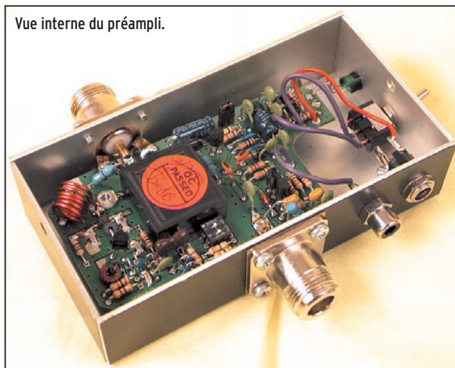
En cas de montage au ras des antennes, prévoir une boîte étanche.
