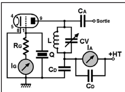
Figure 2: Schéma de l'oscillateur à quartz.
