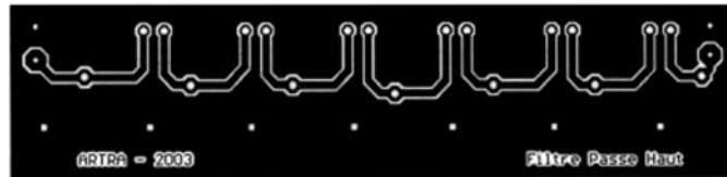
Circuit imprimé du filtre passe haut.
