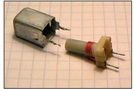
Figure 6: Une petite self et son blindage.
