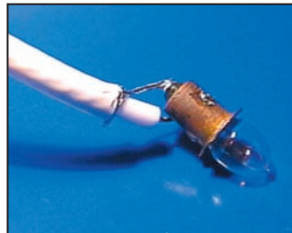
Figure 11: Branchement du câble coaxial sur la charge.
