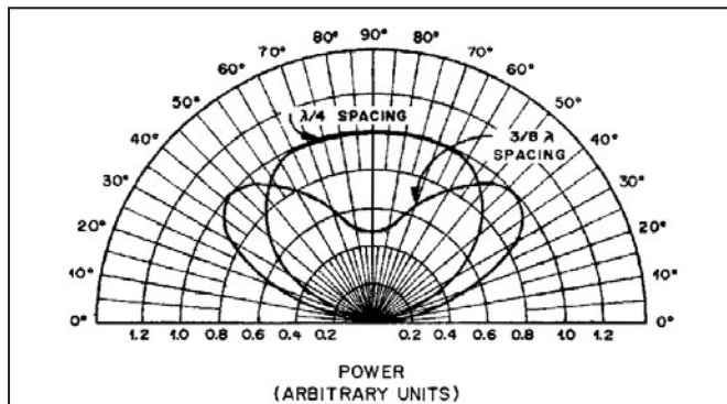
Fig. 10 - Diagramme polaire d'une antenne Turnstile.
