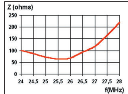
Fig. 6 - Variation de l'impédance en fonction de la fréquence.
