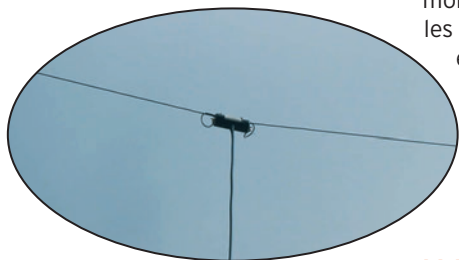
2 - Une vue sur le balun transformateur d'impédance et la descente coaxiale.
