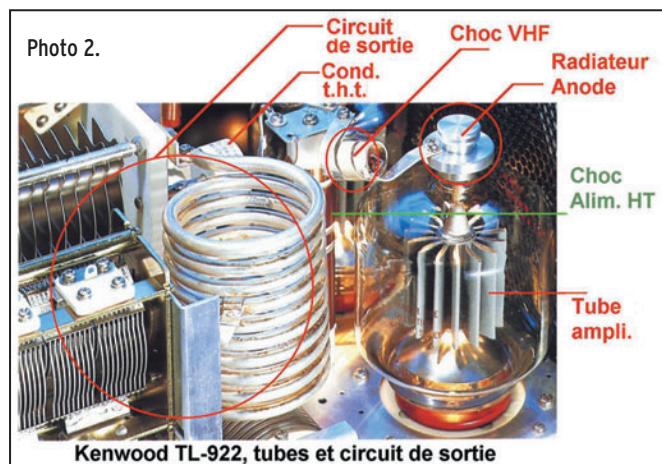
Kenwood TL-922, tubes et circuit de sortie
