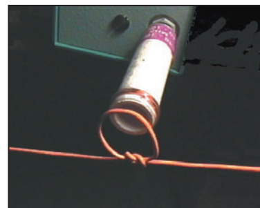
Fig. 2 - Mesure de la fréquence de résonance du dipôle.
