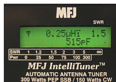
6 - Les valeurs des composants mis en circuit.
