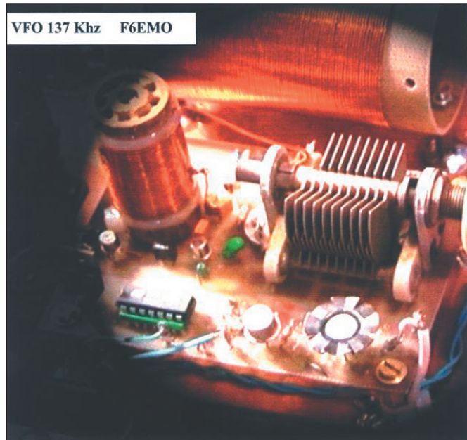
2 - Une vue du VFO.
