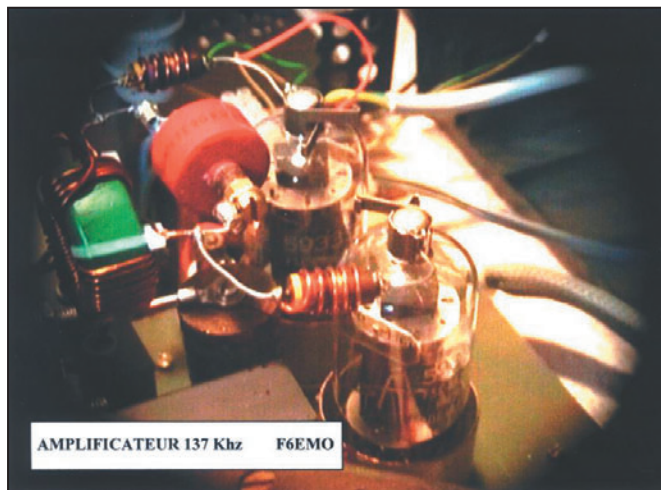
1 - Une vue de l'étage amplificateur 4 watts.
