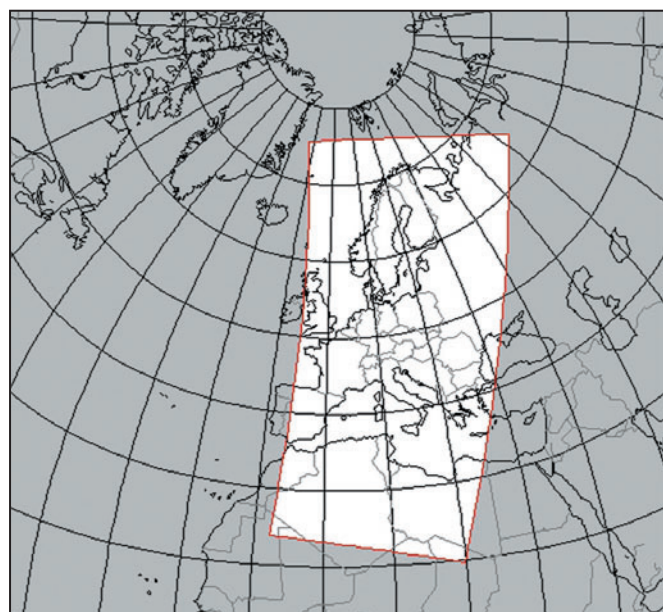
Fig. 1 - Passage sur Europe (POES).
