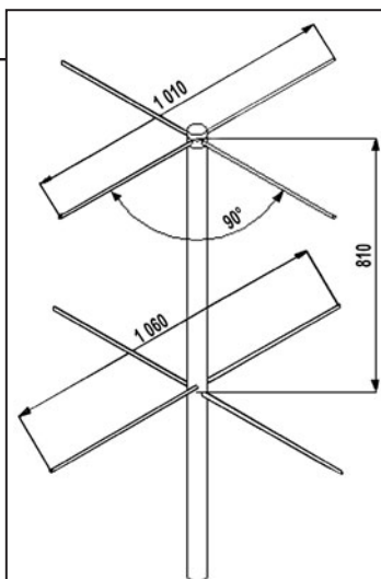
Fig. 8 - Réalisation pratique d'une antenne Turnstile.
