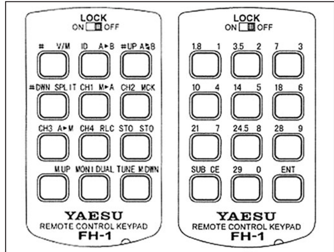
Figure 4 - FH-1: disposition des touches en configuration "keyer" (g.) et "memory" (d.). d'obtenir toutes les fonctions de l'accessoire Yaesu FH-1.
