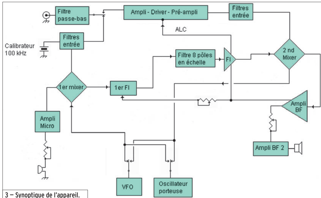
3 - Synoptique de l'appareil.
