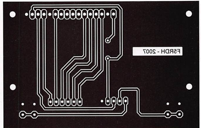
Circuit imprimé de la platine de commande.
