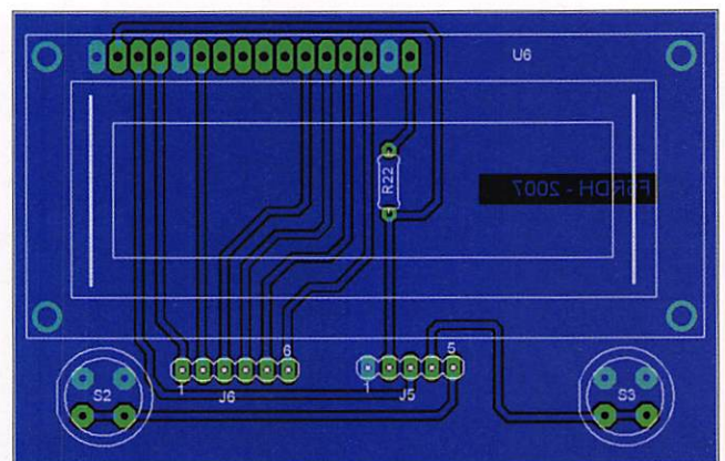
Implantation de la platine de commande.
