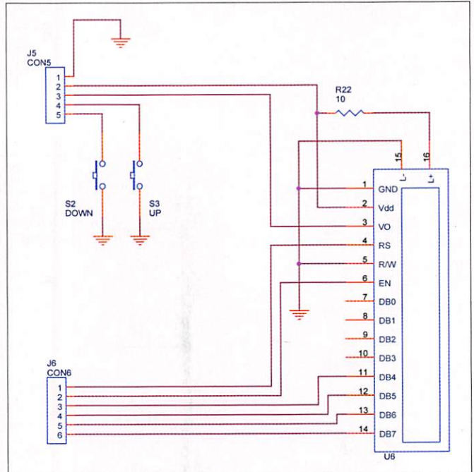
Schéma de principe de la platine de commande.
