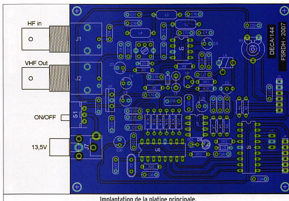
Implantation de la platine principale.
