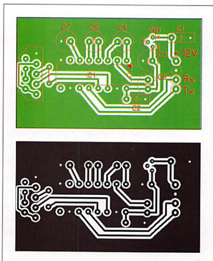
Figure 15A - Implantation composants convertisseur RS232. Figure 15B - CI convertisseur RS232.
