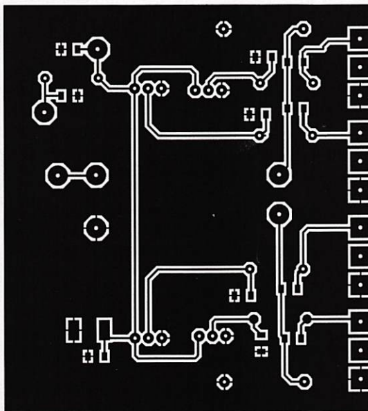
5b - Circuit imprimé circuit de polarisation.
