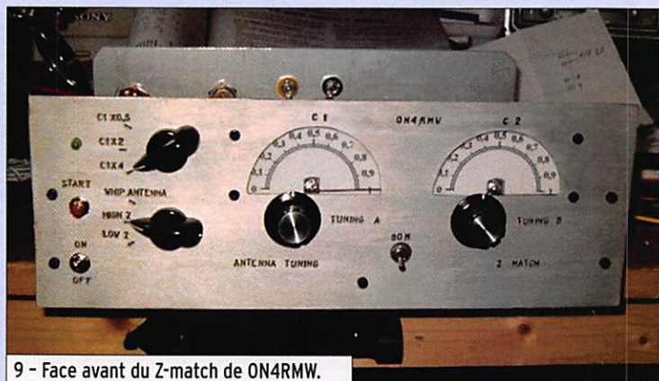
9 - Face avant du Z-match de ON4RMW.
