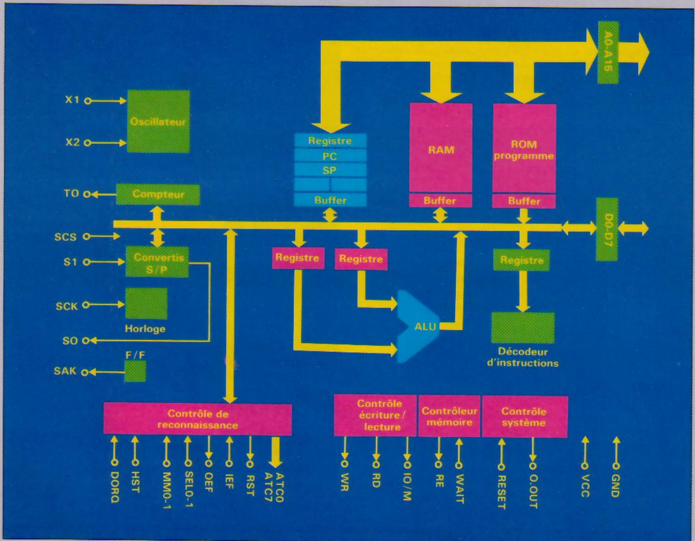
Fig. A. - Synoptique du \mu PD 7762.
