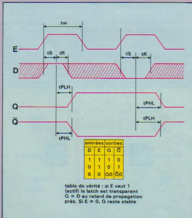
Fig. B. - Diagramme temporel et table de vérité du 74LS75.
