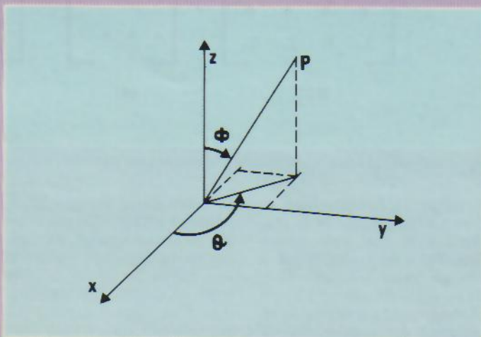
Fig. 1. - Coordonnées sphériques.
