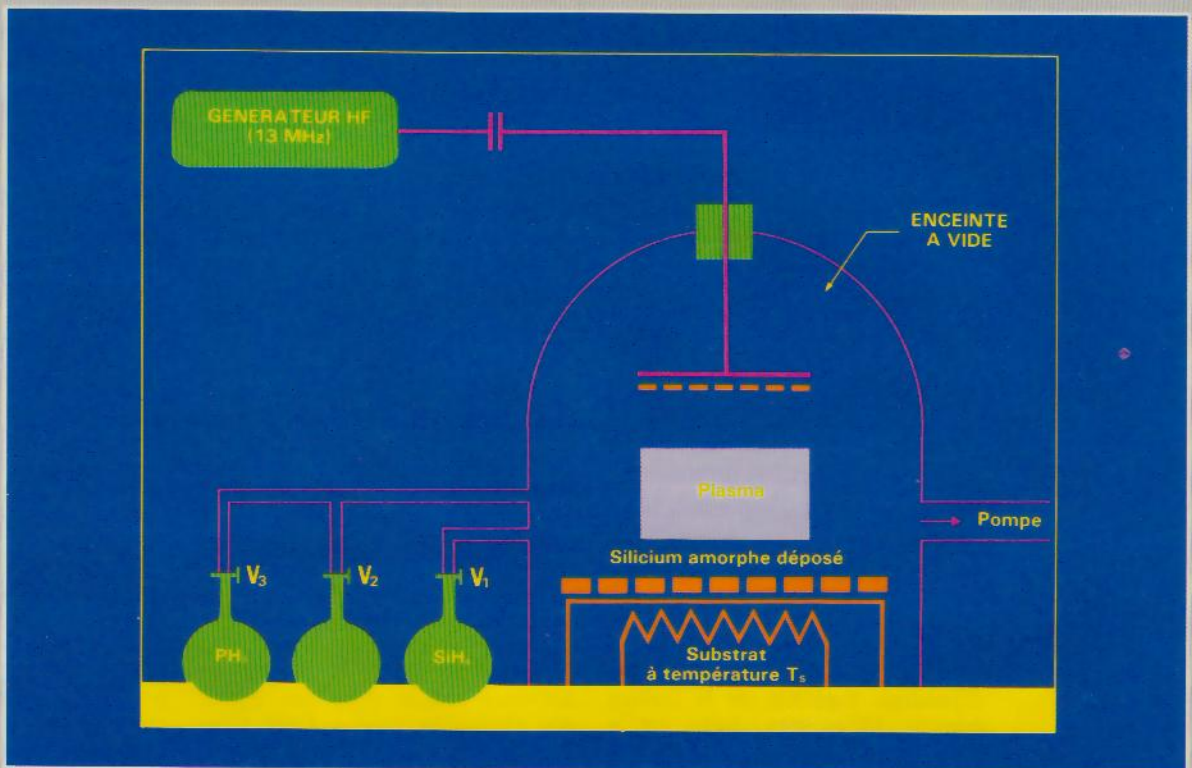
Fig. 9. - Le silicium amorphe hydrogéné ( a\text{-Si:H} ) est obtenu par décomposition de gaz silane sous l'effet d'un champ de haute fréquence. Le plasma formé se dépose sur un substrat maintenu à une température contrôlée T_s = 250^\circ\text{C} . Le dopage se fait en ouvrant, en même temps que la vanne V_1 qui contrôle le débit de silane ( \text{SiH}_4 ), la vanne V_2 pour libérer le diborane ( \text{B}_2\text{H}_6 ) ou la vanne V_3 pour libérer la phosphine ( \text{PH}_3 ), et obtenir ainsi des couches intrinsèques, de type p ou de type n (procédé Solems).
