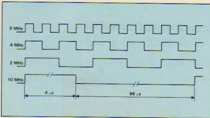
Fig. 3. - Timing des quatre horloges de synchronisation.
