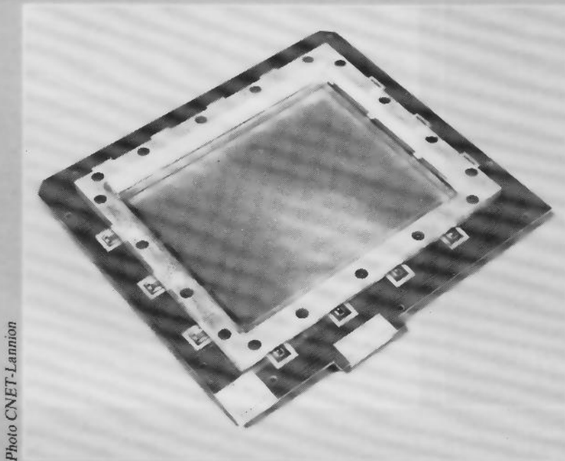
Ecran plat à adressage matriciel par transistors en couche mince au silicium amorphe.
