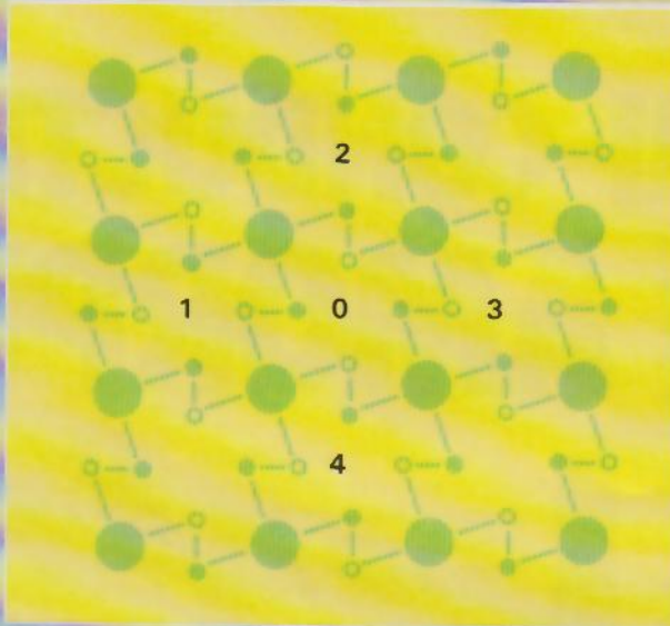
Fig. 1. - Représentation bidimensionnelle d'un cristal de silicium. En réalité, chaque atome se trouve au centre d'un tétraèdre dont les sommets sont occupés par ses quatre voisins. Ainsi l'atome 0 « profite » d'un électron de ses voisins 1, 2, 3 et 4 qui sont mis en commun de manière à saturer sa couche de valence (couche externe) à huit électrons.
