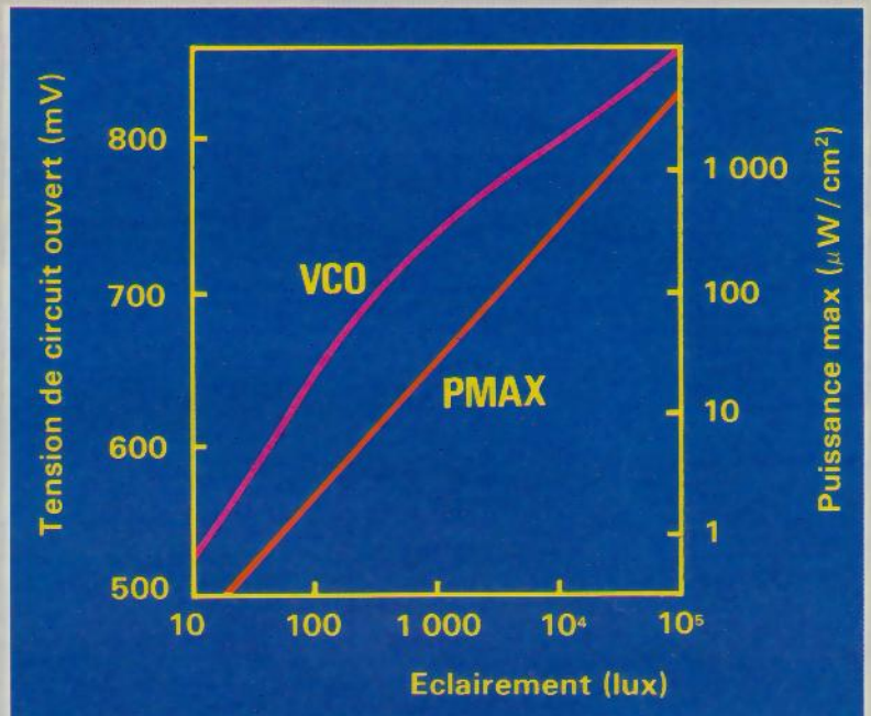
Fig. 14. - Les photopiles au silicium amorphe fonctionnent dans des conditions d'éclairage très différenciées.
