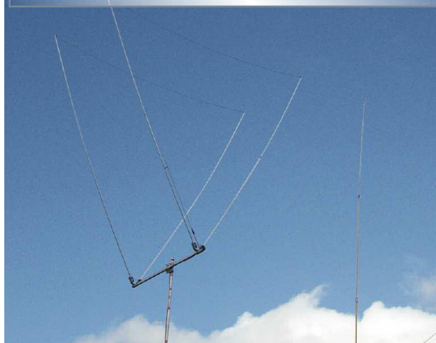
L'antenne 2 éléments DELTA LOOP sur la bande des 10 mètres.
