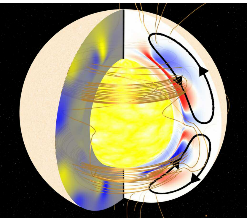
Ci-dessous : vue artistique de la coupe du soleil et de ses différents rayonnements internes. Source NASA.GOV par Andrés Muñoz-Jaramillo de Harvard
