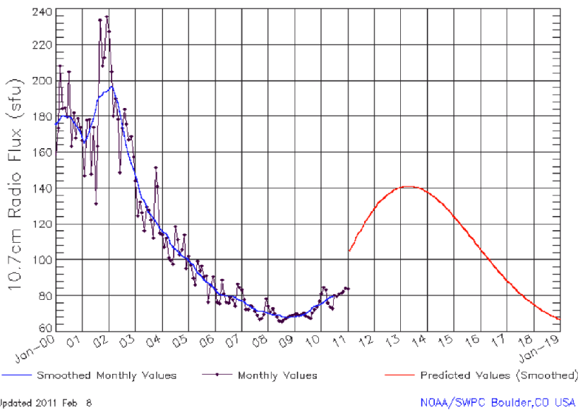
Ci-dessus : graphe du cycle solaire
